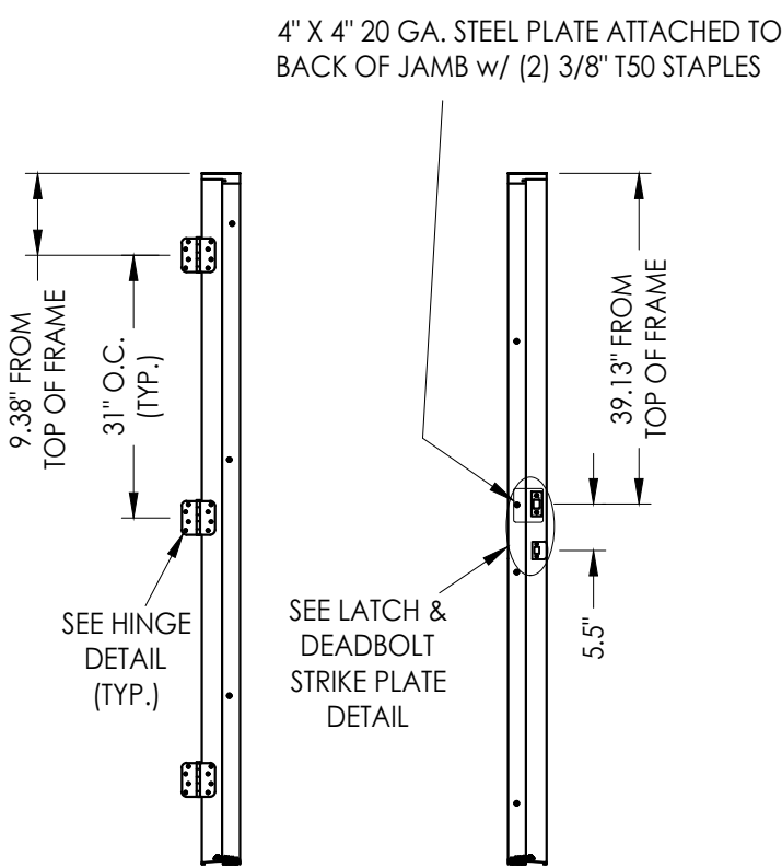
HINGE JAMB
