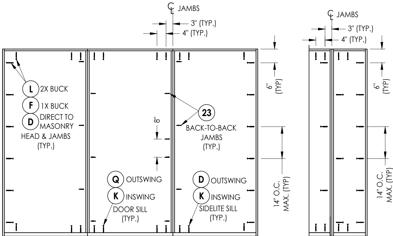
HINGE JAMB
